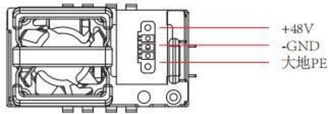
图 3-1 直流电源连接示意图
