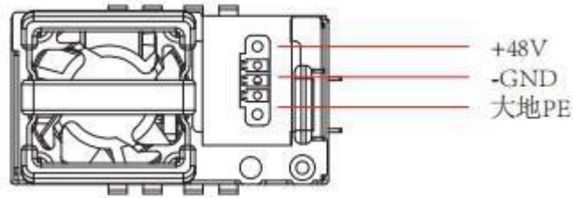
图 1-8 直流电源前面板
